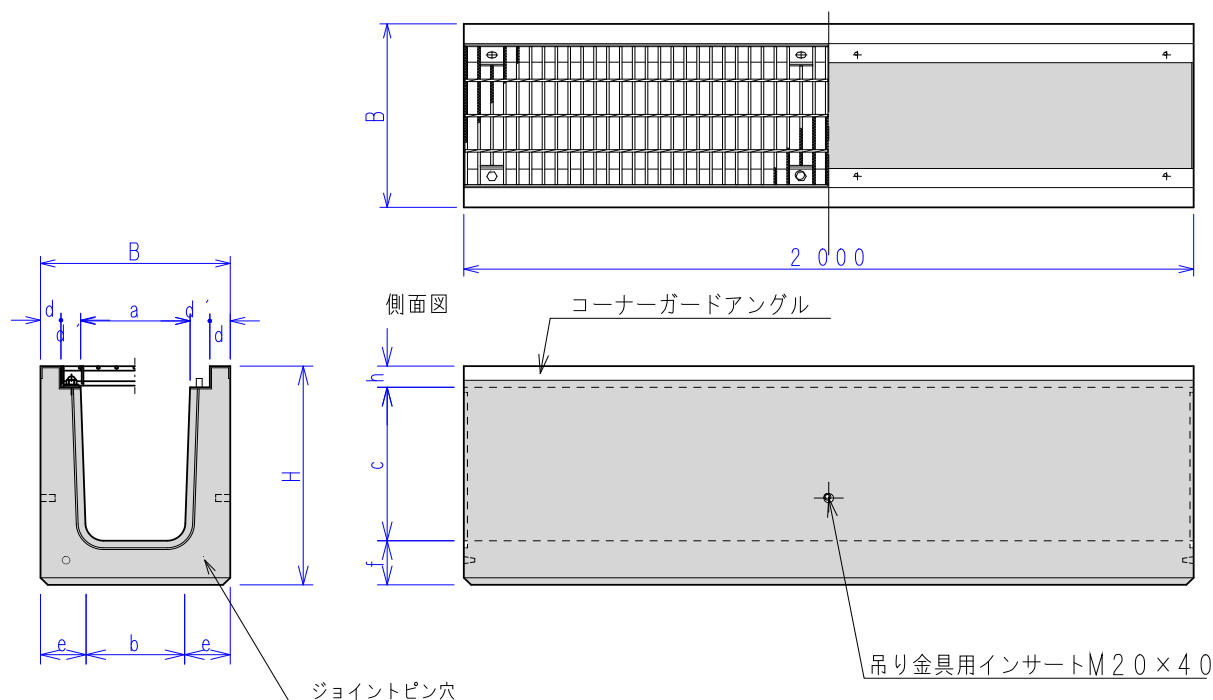
平面図
