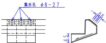
排水ドレン部詳細
